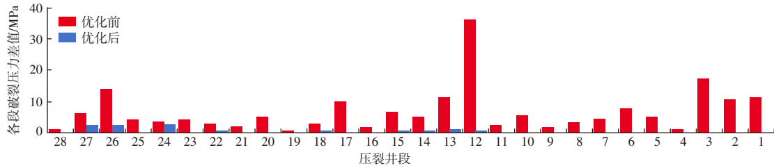
图4 NC1井水平段优化前后破裂压力差值
