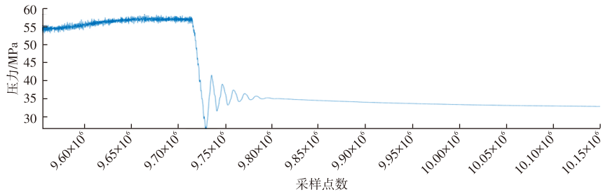
b. 高频压力曲线
