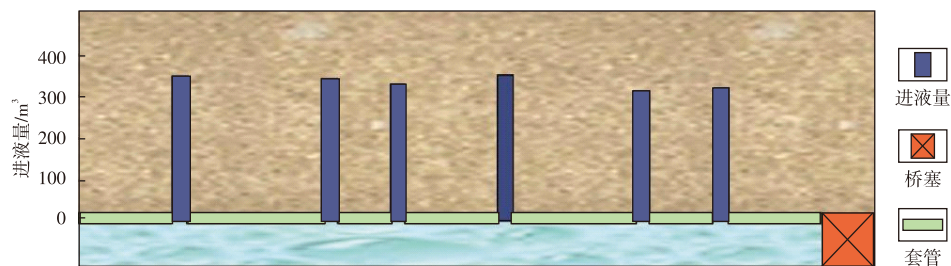
d. NC1井第7段各簇裂缝进液量
