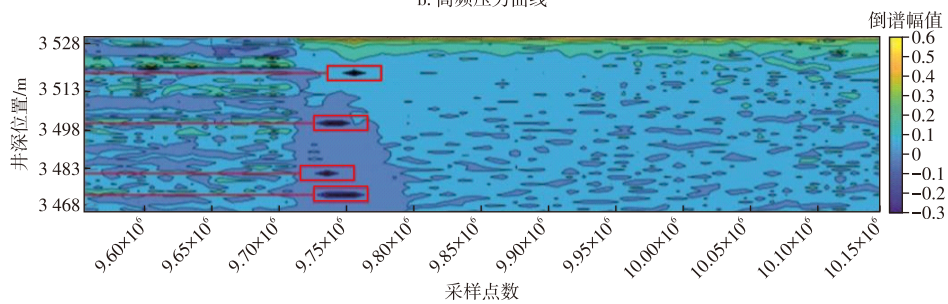
c. 高频压力分析倒谱
