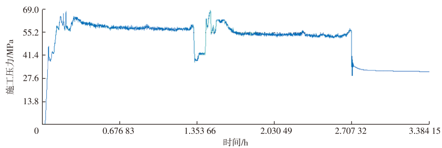
a. 压裂施工压力曲线
