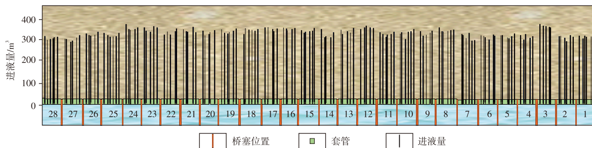
图9 NC1井全井段高频压力倒谱分析反演簇裂缝进液量
